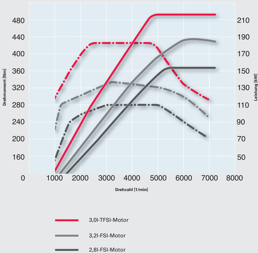
Drehmoment-Leistungskurven der V6-FSI-Motoren
