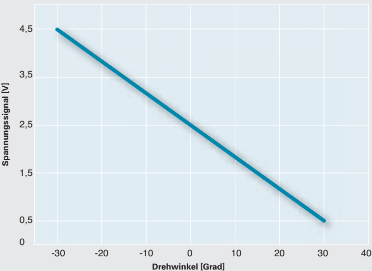
Signalbild des Potenziometers für Saugrohrklappe
